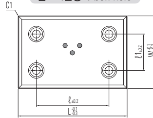
볼트 4홀형 4 bolt hole
