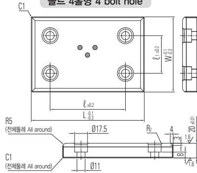
볼트 4홀형 4 bolt hole
