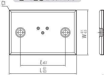
볼트2홀형 2 bolt hole
