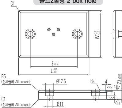
볼트2홀형 2 bolt hole
